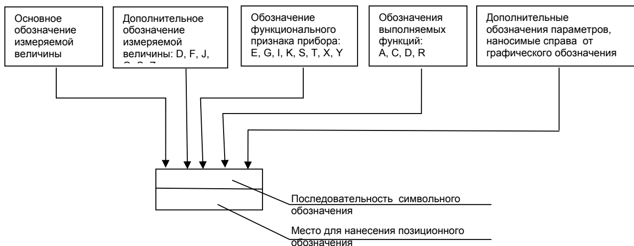
Рисунок 1 - Принцип построения условного обозначения прибора
